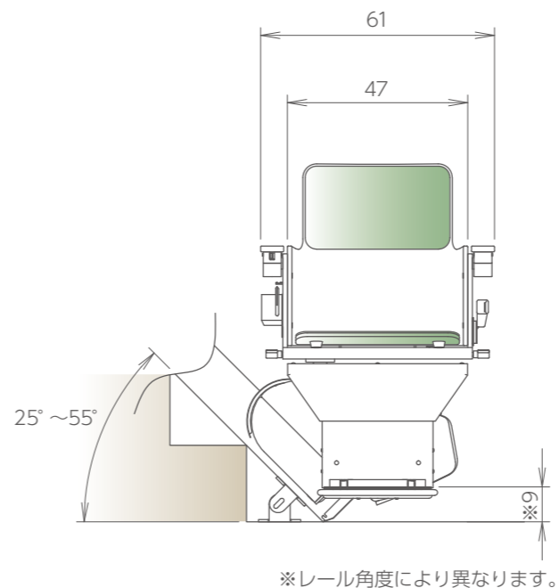
いす正面図
